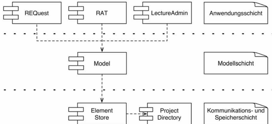
Abb. 3: Schichtenarchitektur von Sysiphus (UML Komponentendiagramm)
